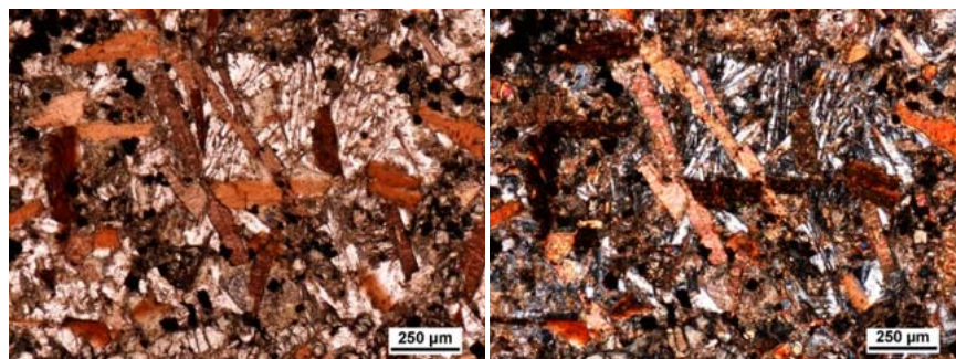
Obr. ke článku: Kersantit ve spilitu, kamenolom Mítov na Plzeňsku na str. 45 Foto 1. Mikrofotografie kersantitu z kamenolomu Mítov, bez analyzátoru. Autor snímku dr. Štěpánka Mrázová, výbrus Daniela Borovská. Foto 2. Mikrofotografie kersantitu z kamenolomu Mítov, zkřížené nikoly. Autor snímku dr. Štěpánka Mrázová, výbrus Daniela Borovská.
